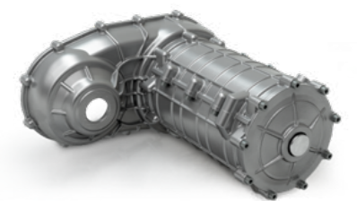
↑ Segmentiertes E-Motorengehäuse
